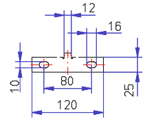
Ansicht "Y"
